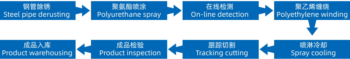
生产工艺流程
